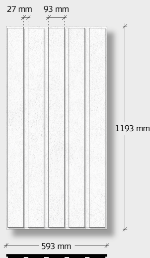
Troldtekt® Tiles 5, T24 25 x 593 x 1193 mm
